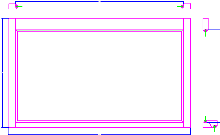
UPPER SASH ELEVATION QTY: 1
